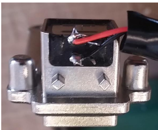
Lodning af ledning til opladerindgang
