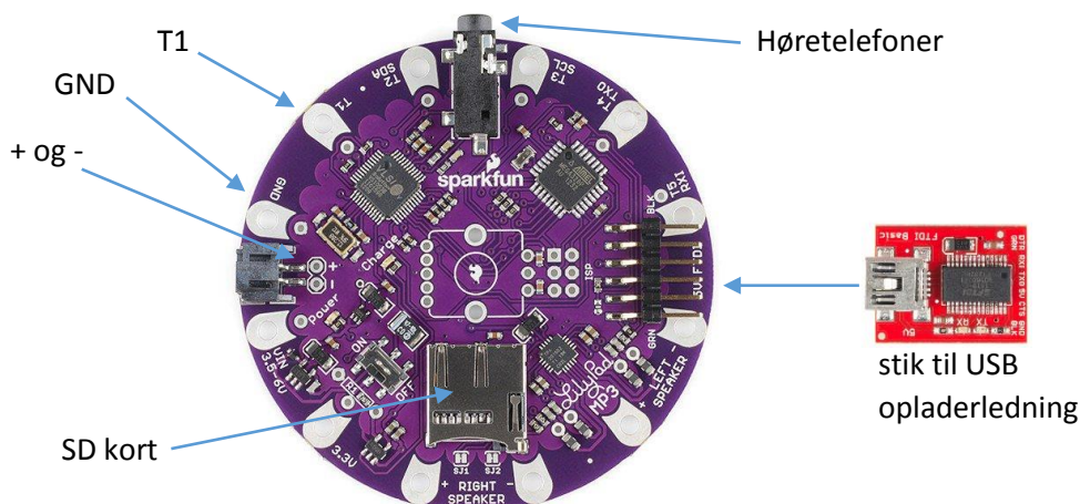
Lodning af ledning til opladerindgang
